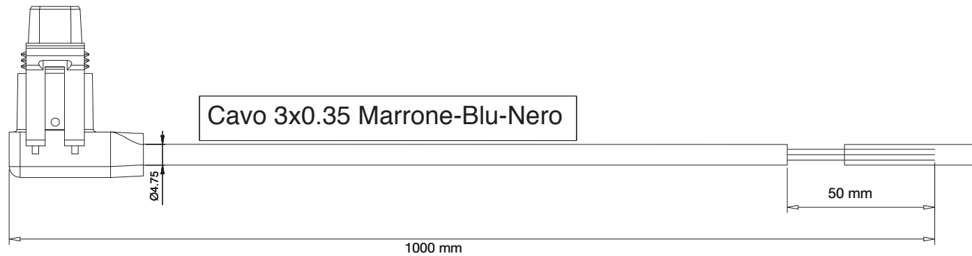
Serie connettore PWSA
