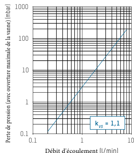
Diagrammes de pertes de pression
